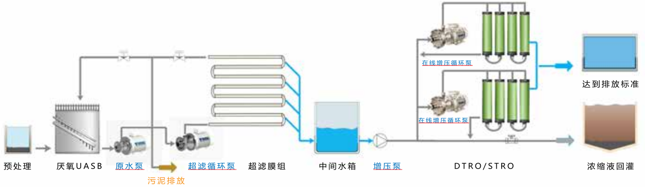
工艺流程图
